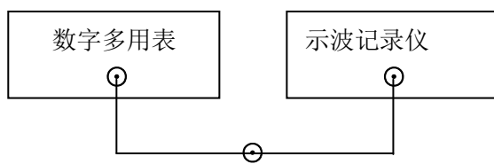
图 2 输入电阻校准连线图
