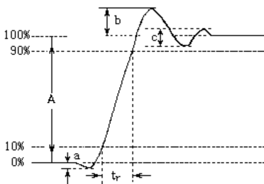
图 4 示波记录仪阶跃响应特性示意图
