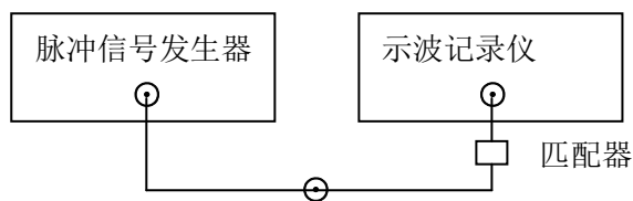
图 9 示波记录仪直流增益校准连线图
