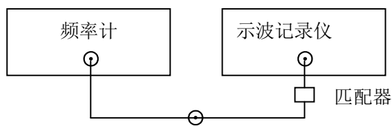
图 6 示波记录仪时基测量校准连线图
