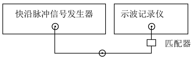
图 3 瞬态特性校准连线图
