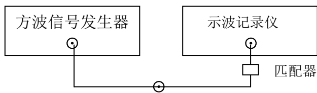
图 11 示波记录仪幅度校准连线图
