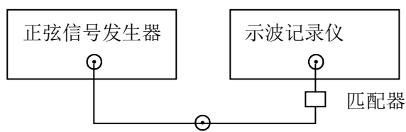
图 12 示波记录仪校准连线图
