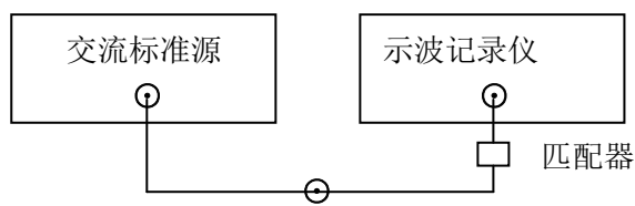
图 10 示波记录仪直流增益校准连线图
