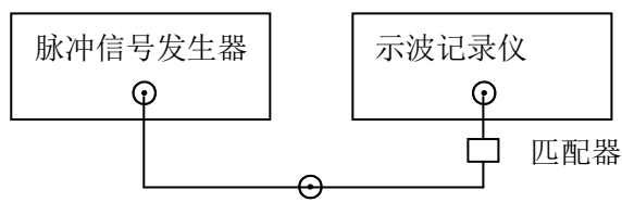
图 7 示波记录仪时间测量校准连线图
